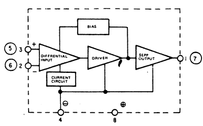
M54565P (Mitsubishi)
