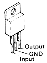
NJM78M24A (JRC)
